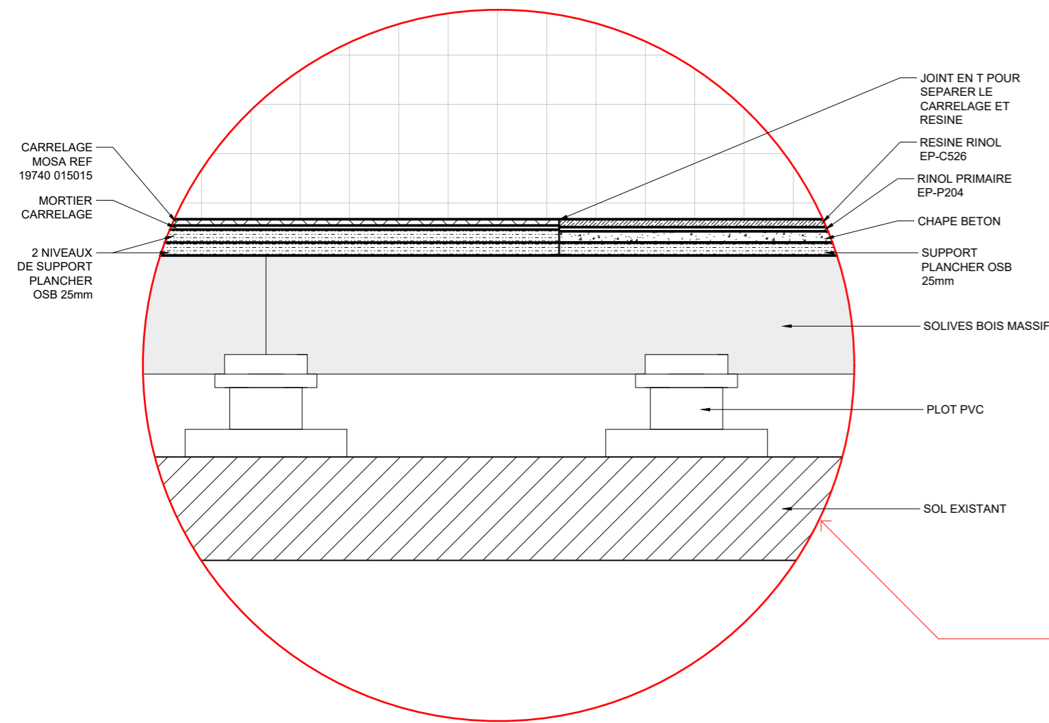
DÉTAIL PLANCHER ÉCHELLE 1:10
